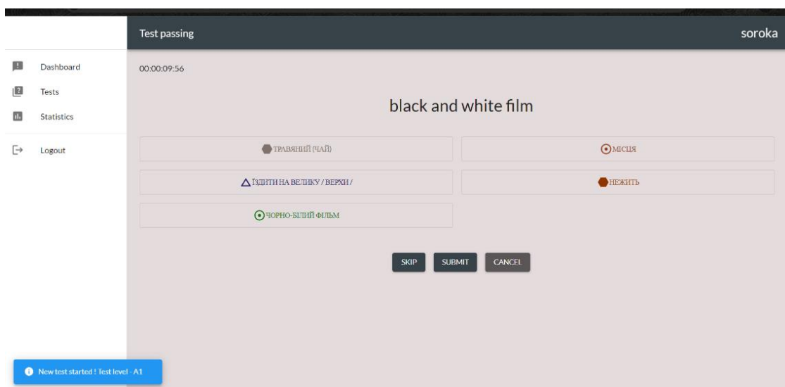
Рис.1. Інтерфейс тесту
