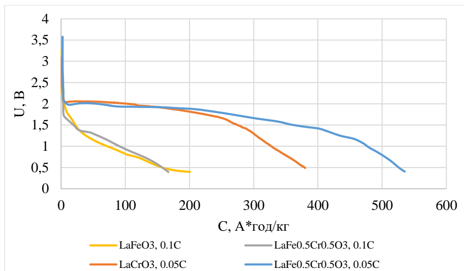
Рис. 2. Розрядна крива отримана в гальваностатичному режимі.
