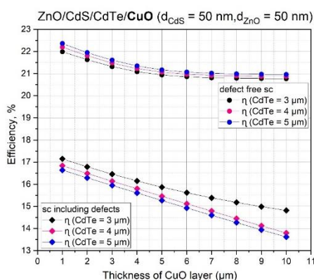
Рис. 1. Зміна величини ефективності \eta для гетеропереходу ZnO/CdS/CdTe/CuO як функції товщини контактної шару CuO ( d_{CuO}=1-10 \mu m ).
