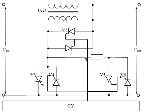
Рис. 1. Схема пристрою з «м'якою» комутацією тиристорів
