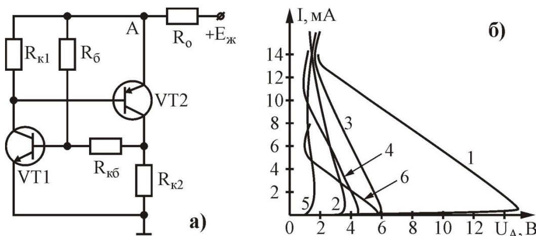
Рис. 1. Схема пристрою із від'ємним диференційним опором (а) та його ВАХ (б) для значень резисторів, указаних у табл. 1
