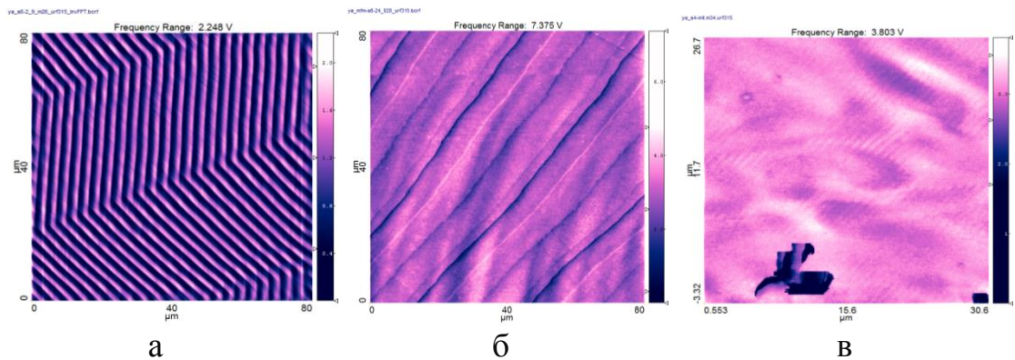
Рис. 1. MFM зображення плівок ЗПГ ( Y_3Fe_5O_{12} ) товщиною 2,9 мкм (а) та 24 мкм (б) та La:ЗПГ ( Y_{2,8}La_{0,2}Fe_{4,2}Ga_{0,8}O_{12} )
