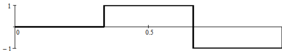
Рис. 1 Графічне подання материнського трійкового симетричного вейвлета
